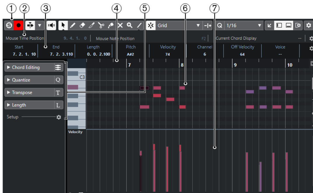
Окно Клавишный редактор в нижней зоне окна Проект :
