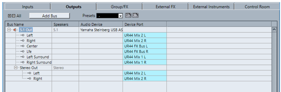
Bus de salida en configuración de canales 5.1 con un subbus estéreo
