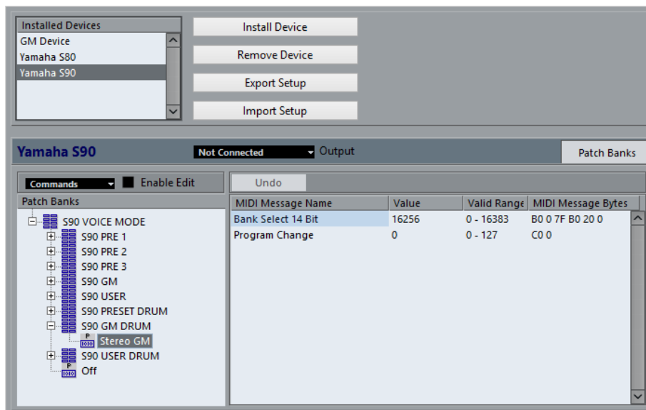
Менеджер MIDI устройств в Cubase Artist.
