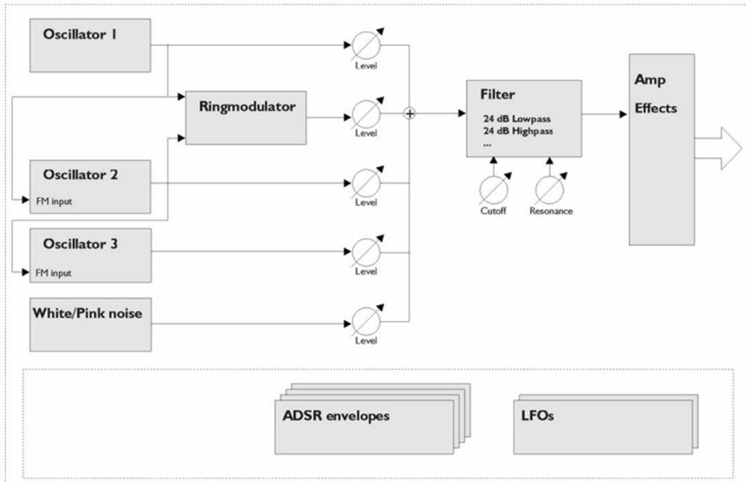
Функциональная диаграмма
