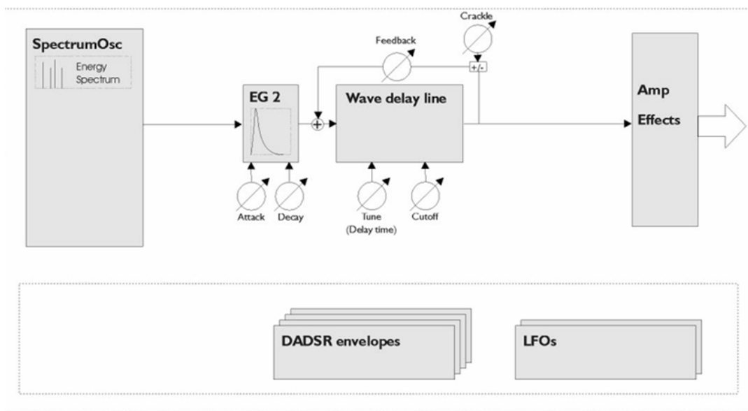
Функциональная диаграмма
