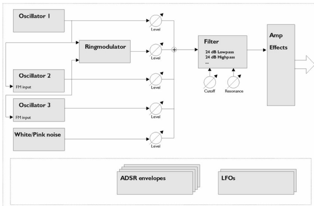
Функциональная диаграмма
