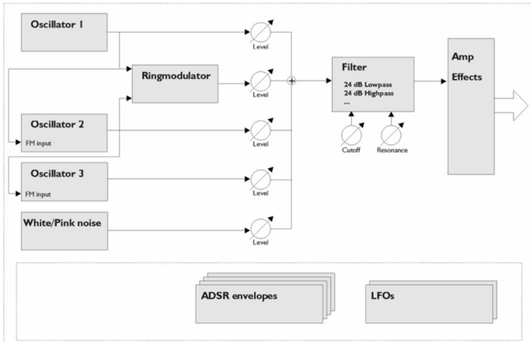
Diagrama funcional
