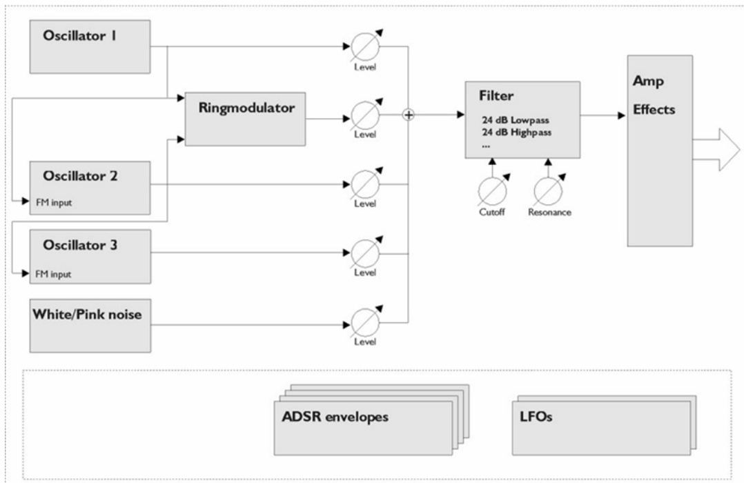
Schémas fonctionnels
