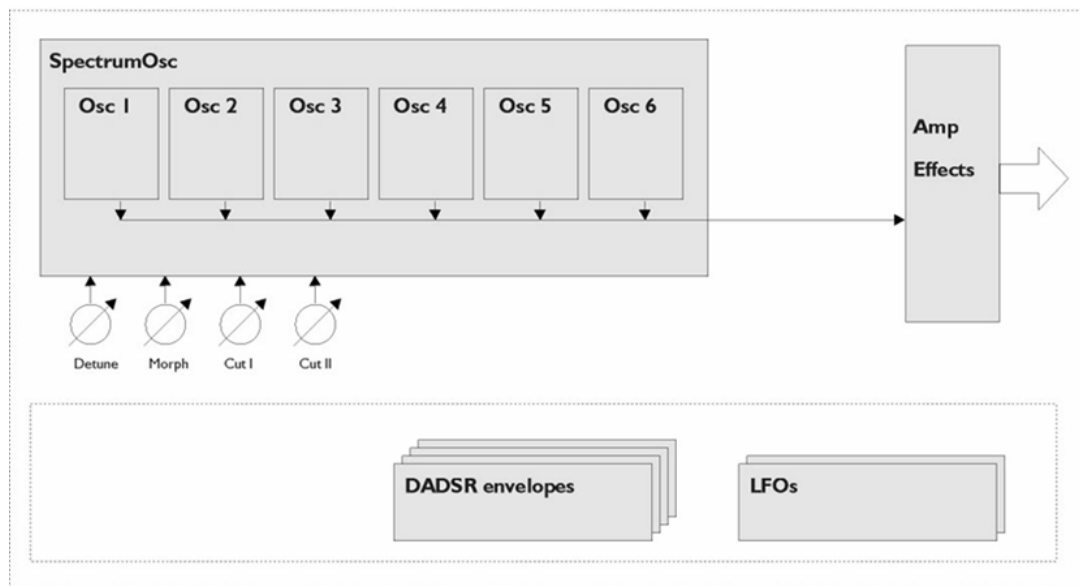
Diagrama funcional
