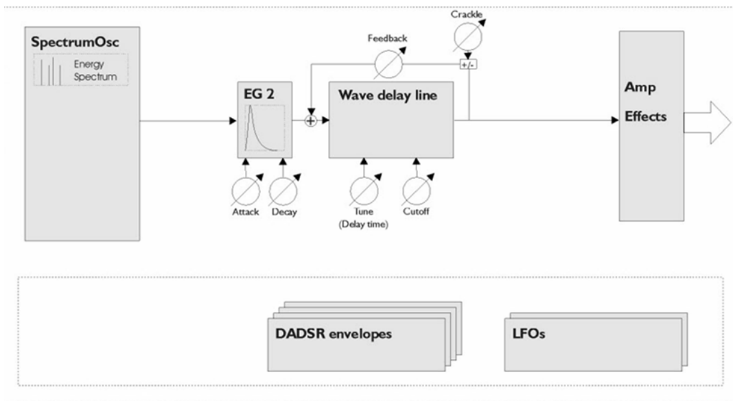
Функциональная диаграмма
