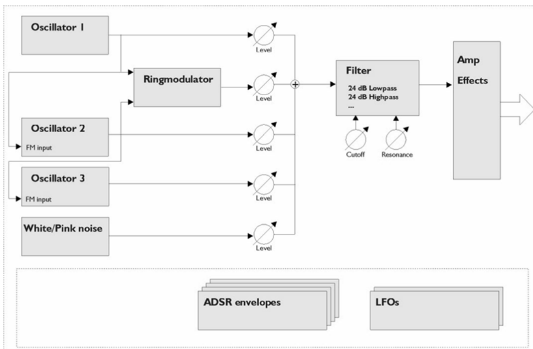
Функциональная диаграмма
