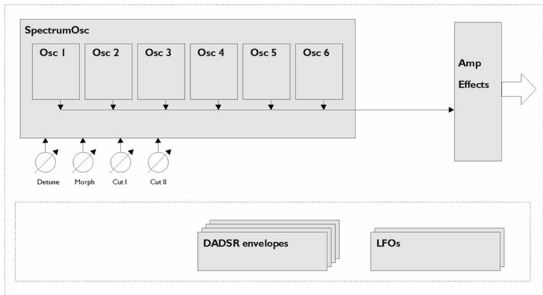
Schémas fonctionnels
