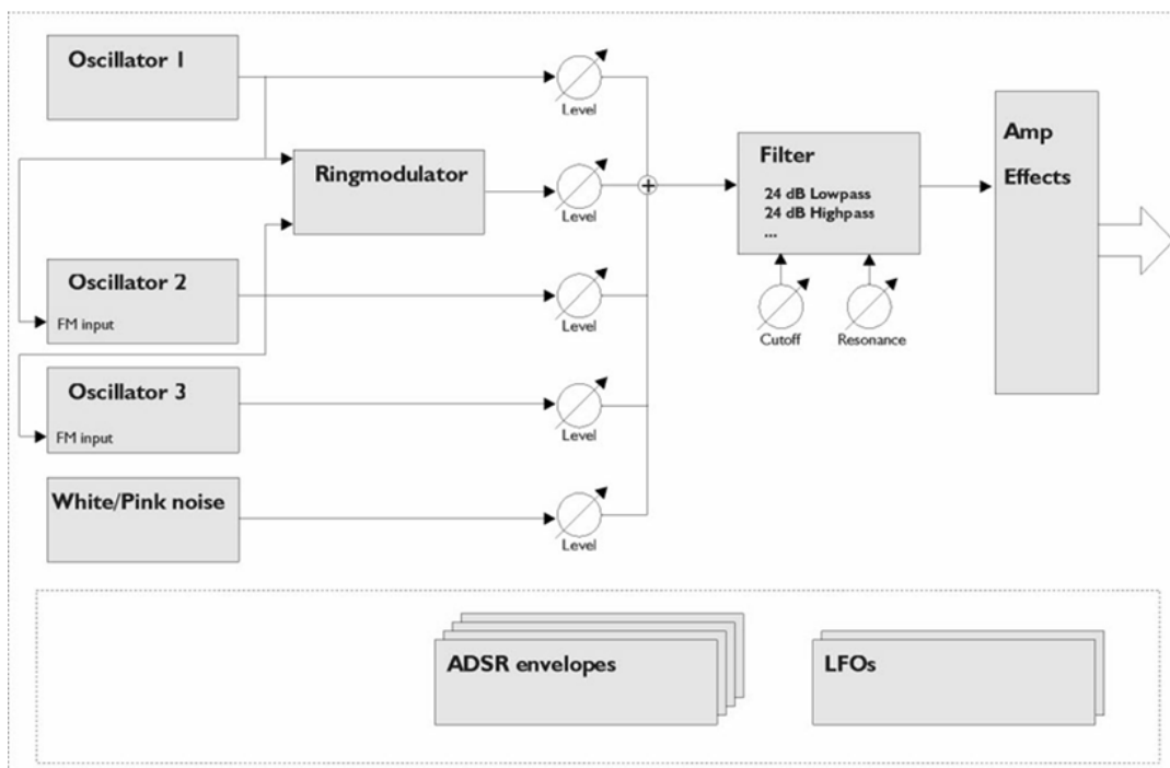
Функциональная диаграмма
