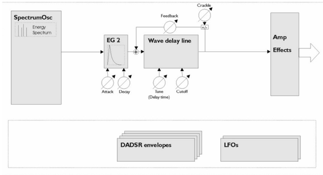
Функциональная диаграмма
