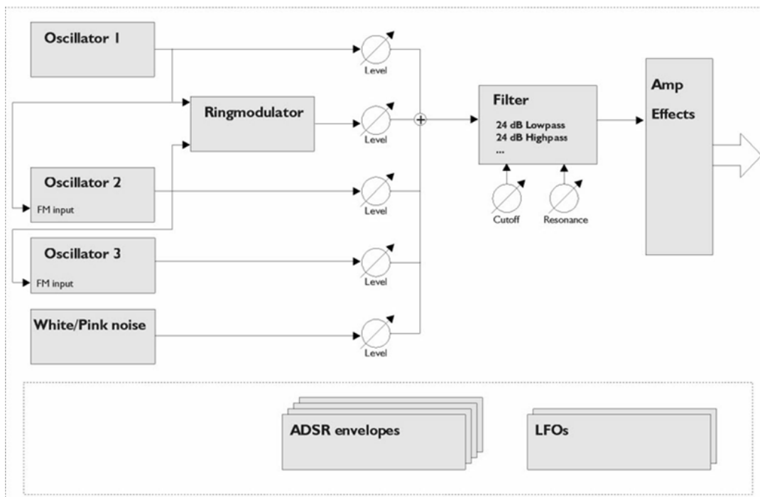
Schema funzionale
