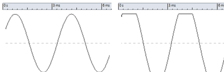
Forme d'onde sinusoïdale avant et après écèlement.
